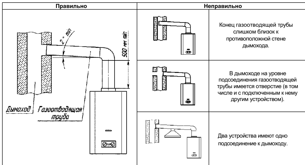
Рисунок 9. Подключение аппарата к дымоходу
